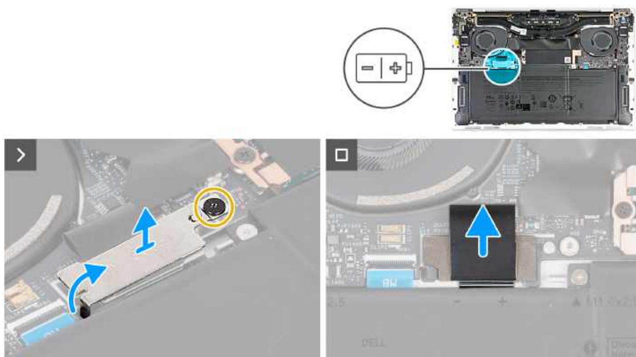
Rysunek 13. Wymontowywanie pokrywy dolnej
