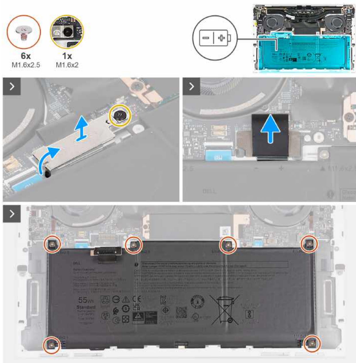
Rysunek 17. Wymontowywanie baterii
