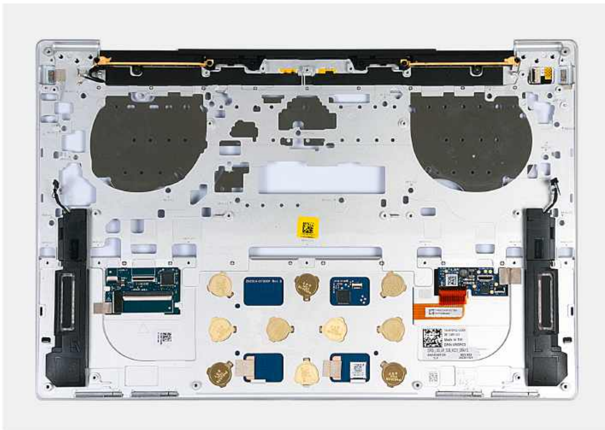
Rysunek 61. Wymontowywanie zestawu podpórki na nadgarstek
