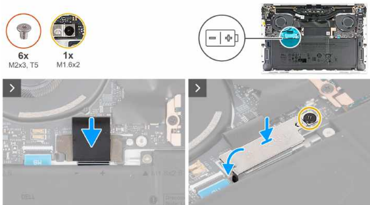
Rysunek 14. Instalowanie pokrywy dolnej
