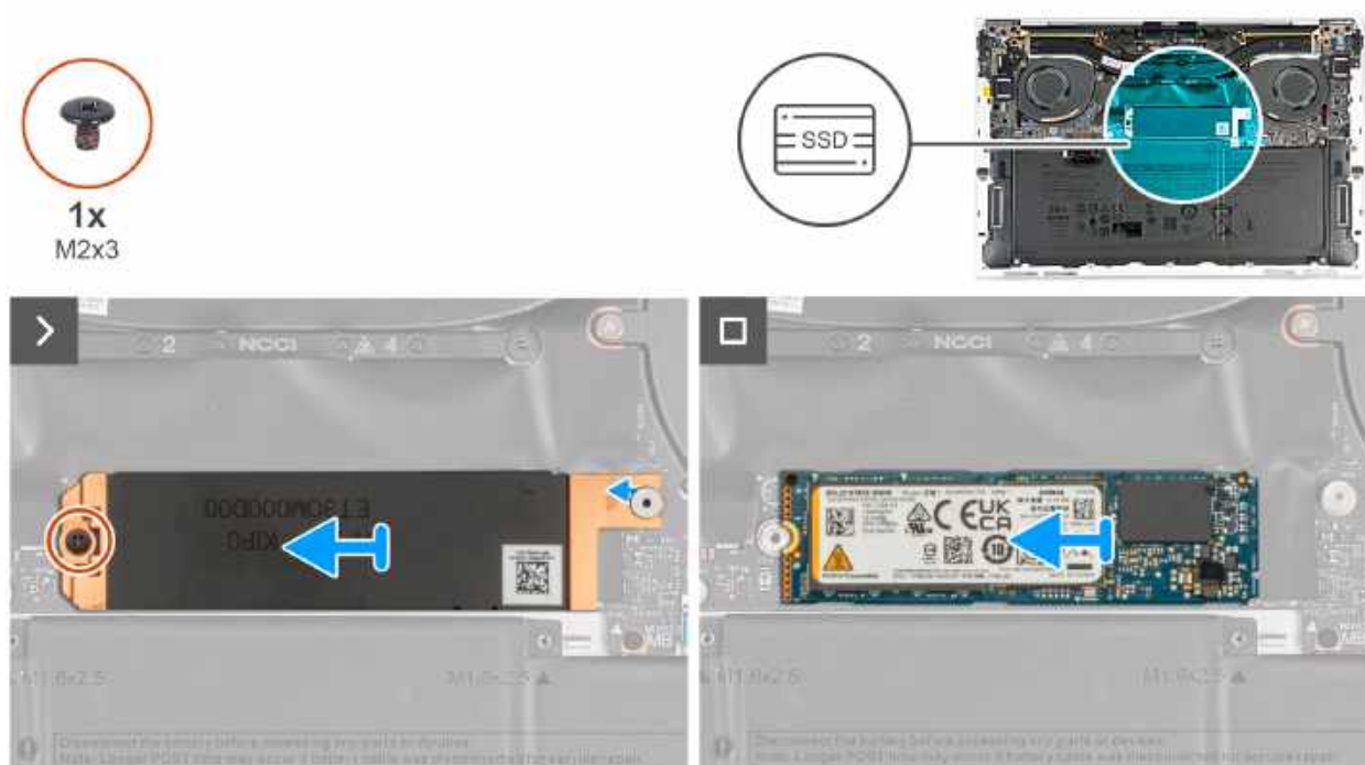
Rysunek 31. Wymontowywanie dysku SSD M.2 2280
