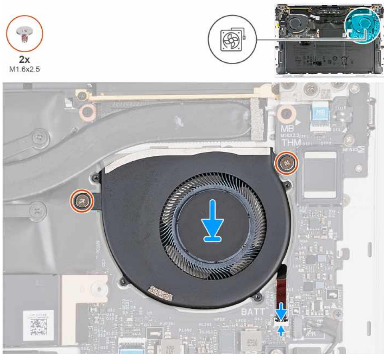
Rysunek 38. Instalowanie lewego wentylatora
