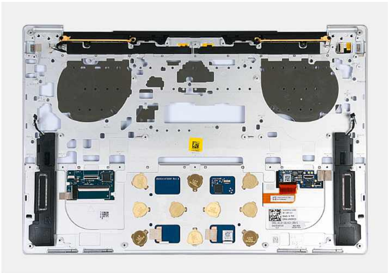
Rysunek 62. Instalowanie zestawu podpórki na nadgarstek
