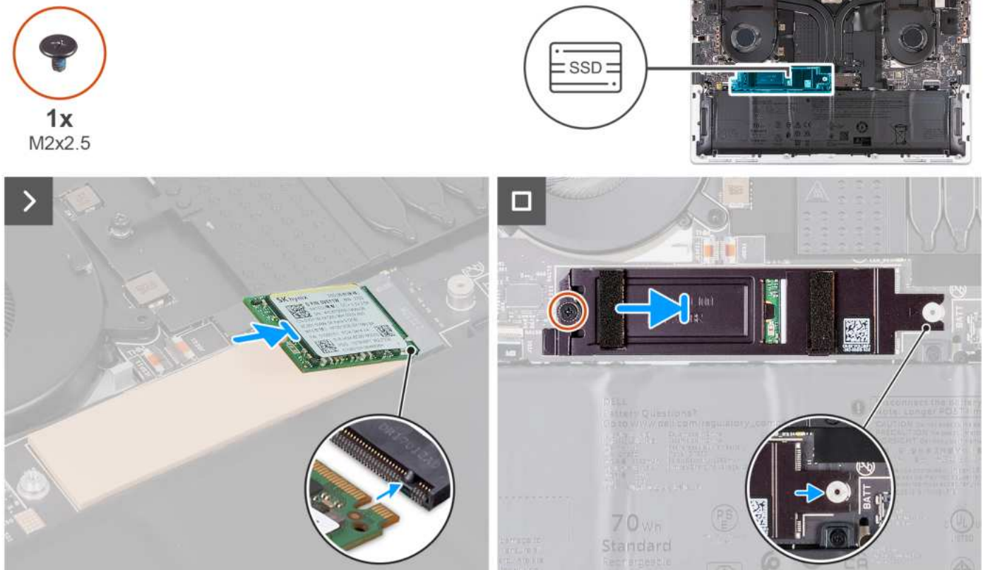
Rysunek 21. Instalowanie dysku SSD M.2 2230
