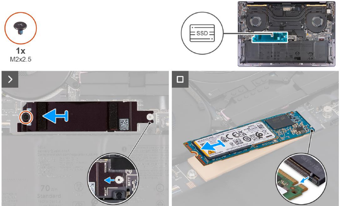
Rysunek 22. Wymontowywanie dysku SSD M.2 2280
