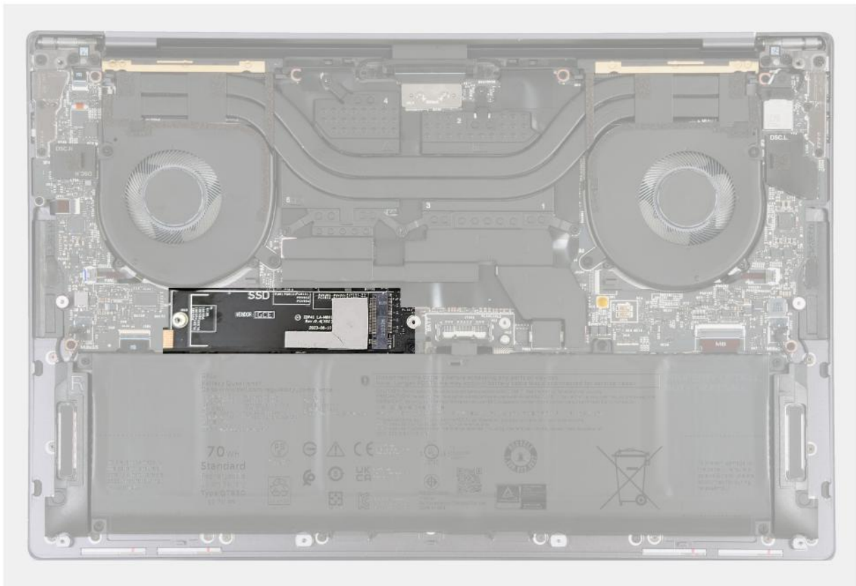
Rysunek 20. Podkładka termoprzewodząca dysku SSD M.2
