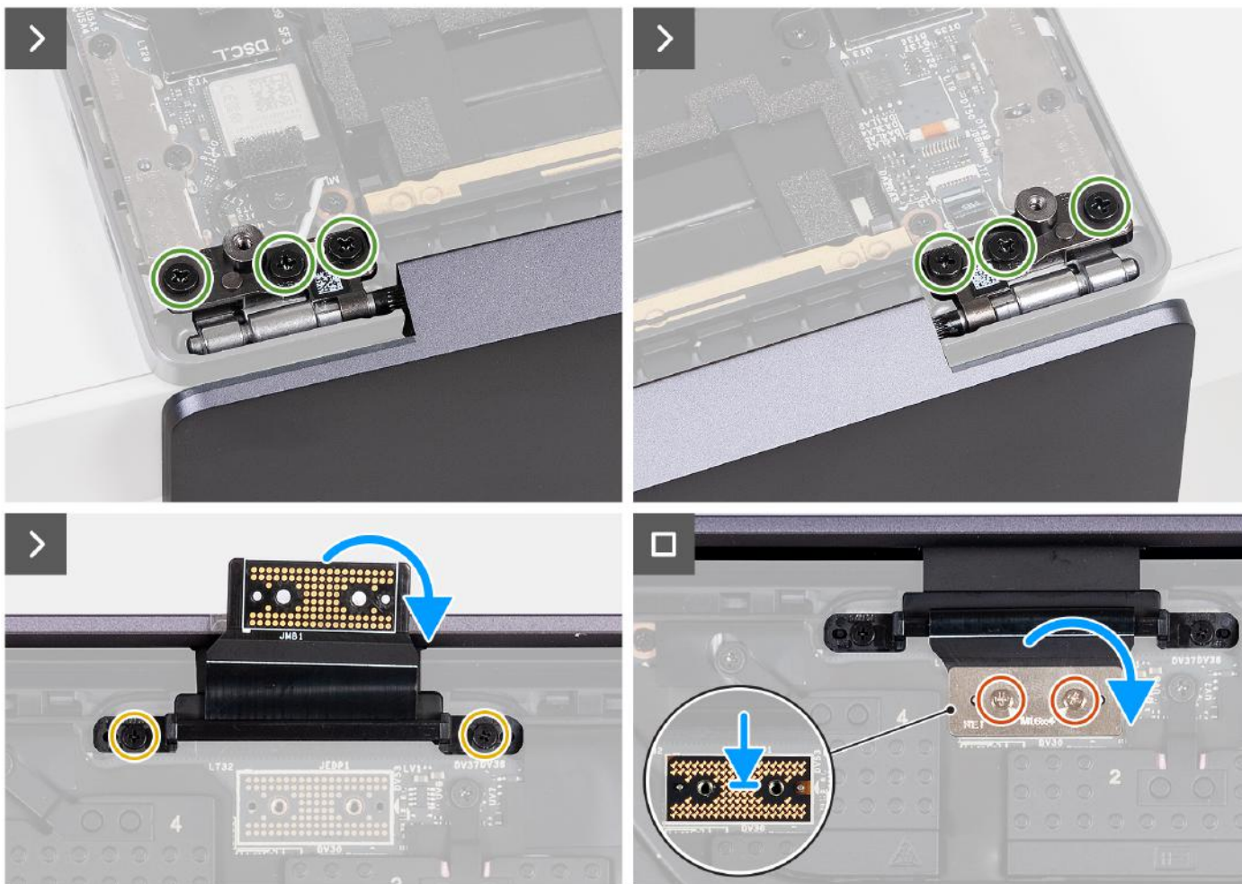
Rysunek 31. Instalowanie zestawu wyświetlacza
