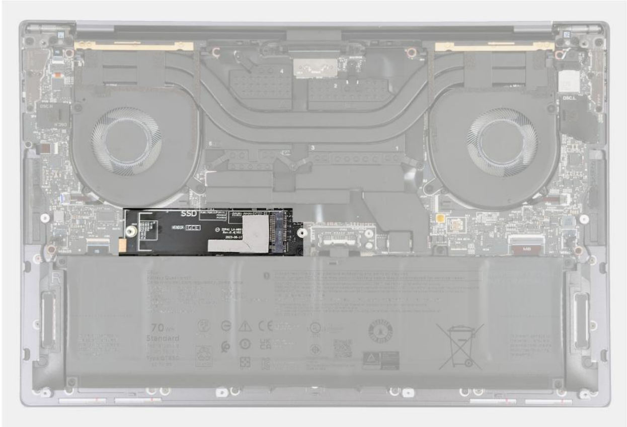
Rysunek 23. Podkładka termoprzewodząca dysku SSD M.2
