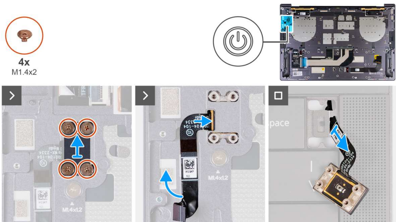
Rysunek 38. Wymontowywanie przycisku zasilania z czytnikiem linii papilarnych
