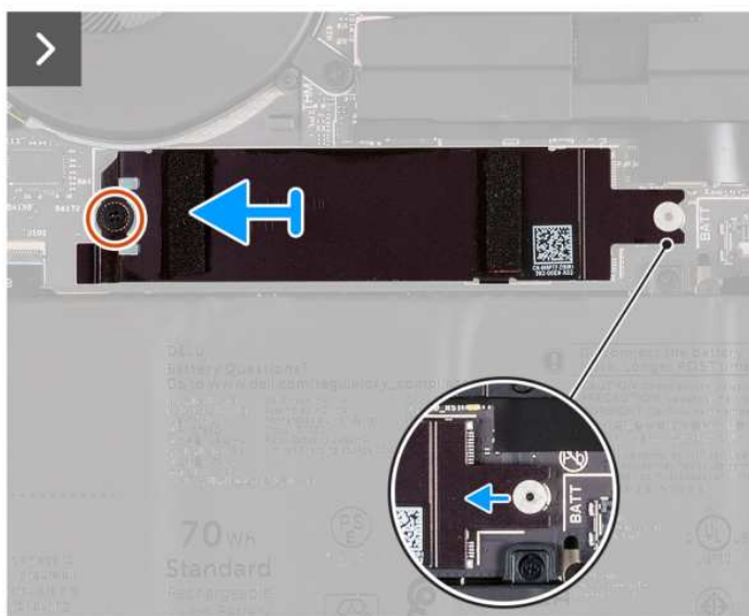
Rysunek 22. Wymontowywanie dysku SSD M.2 2280
