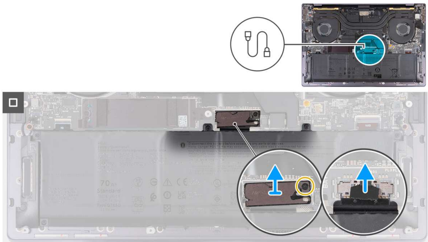
Rysunek 12. Odłączenie kabla baterii od płyty głównej
