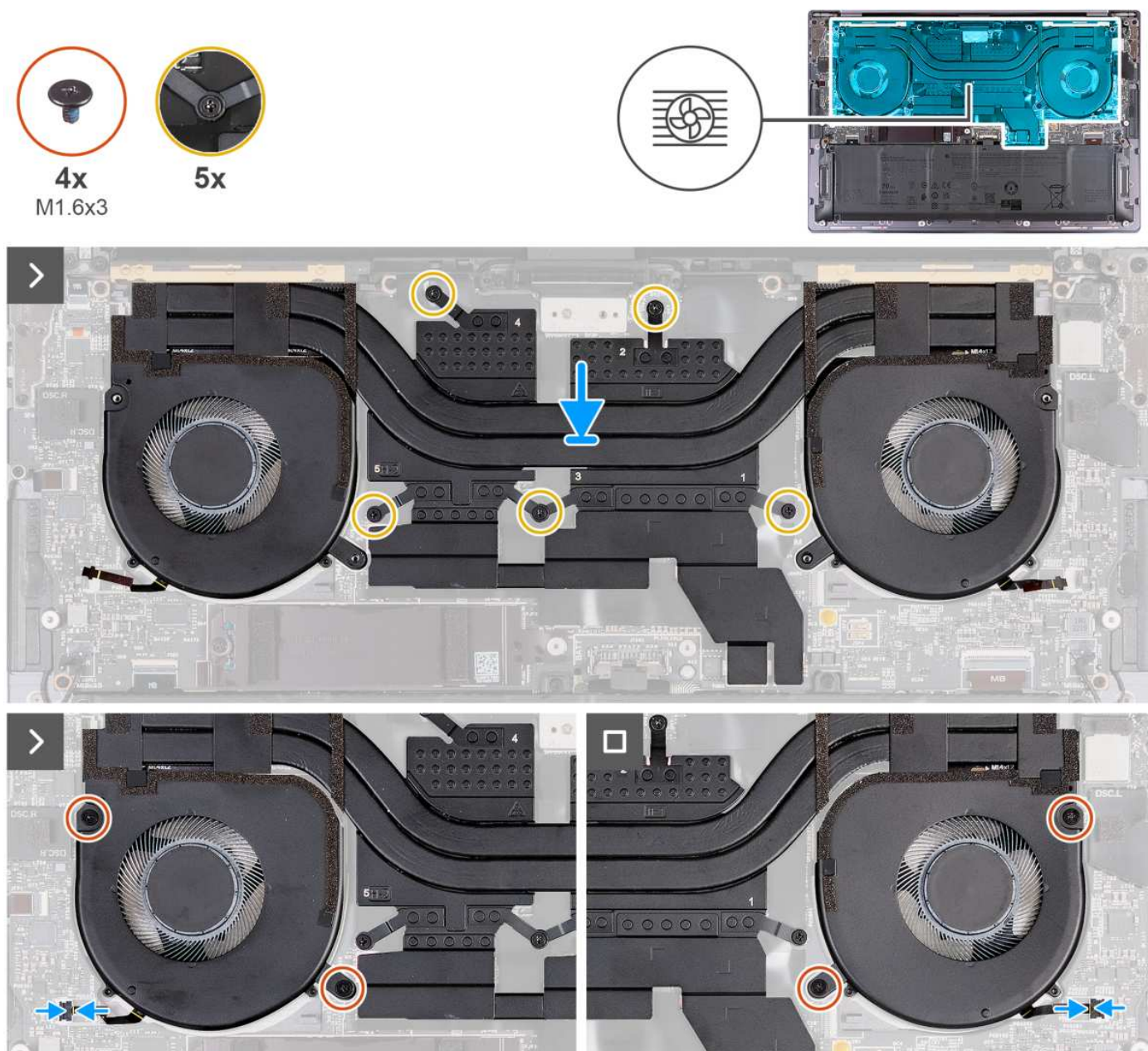
Rysunek 26. Instalowanie zestawu radiatora
