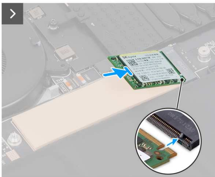
Rysunek 21. Instalowanie dysku SSD M.2 2230
