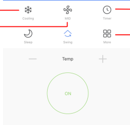
GLÓWNY INTERFEJS
