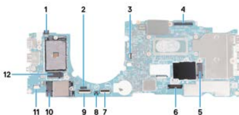
Rysunek 8. Złącza na płycie głównej
