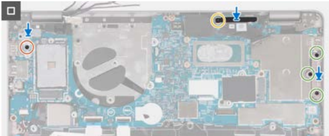
Rysunek 11. Instalowanie płyty głównej
