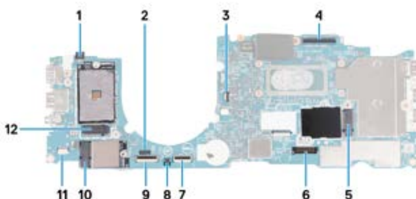
Rysunek 4. Złącza na płycie głównej
