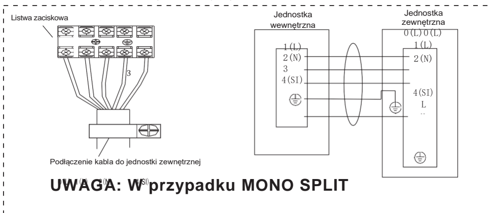
Podłączenie kabla do jednostki zewnętrznej
