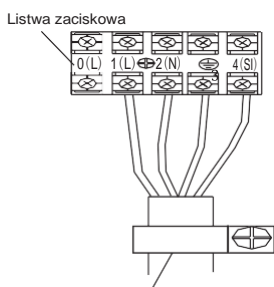
Podłączenie kabla do jednostki zewnętrznej
