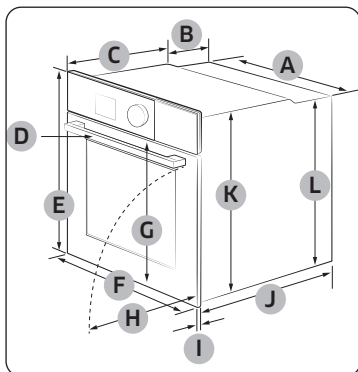
Piekarnik (mm)
