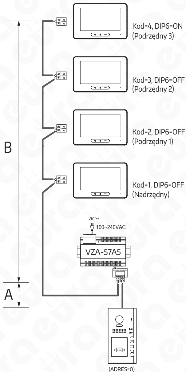
Rys. 10. Schemat rozbudowy przykładowego zestawu z kasetą VZA-57A5 o dodatkowe monitory oraz dobór długości i przekroju przewodów w systemie Eura 2 Easy
